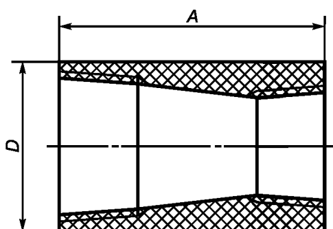
Рисунок 2 — Переходная муфта
